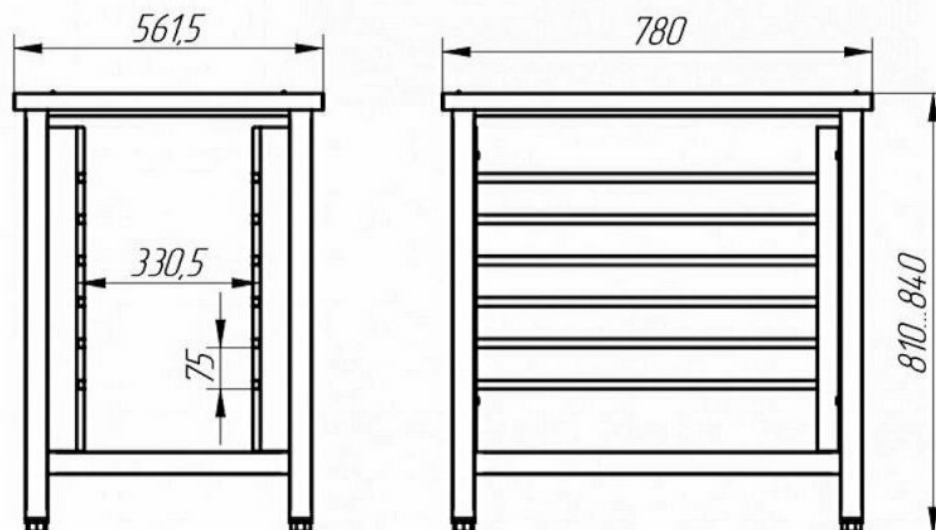
Подставка ПК-6-2/3 под пароконвектомат ПКА6-2/3
