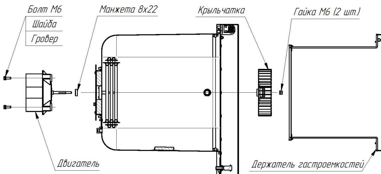
Рис.8. Схема замена манжет.
