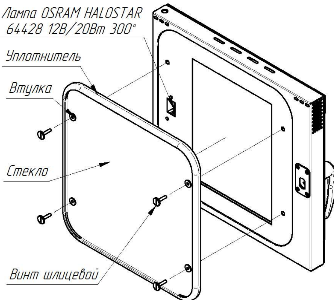
Рис.7. Замена лампы освещения и уплотнителя двери.
