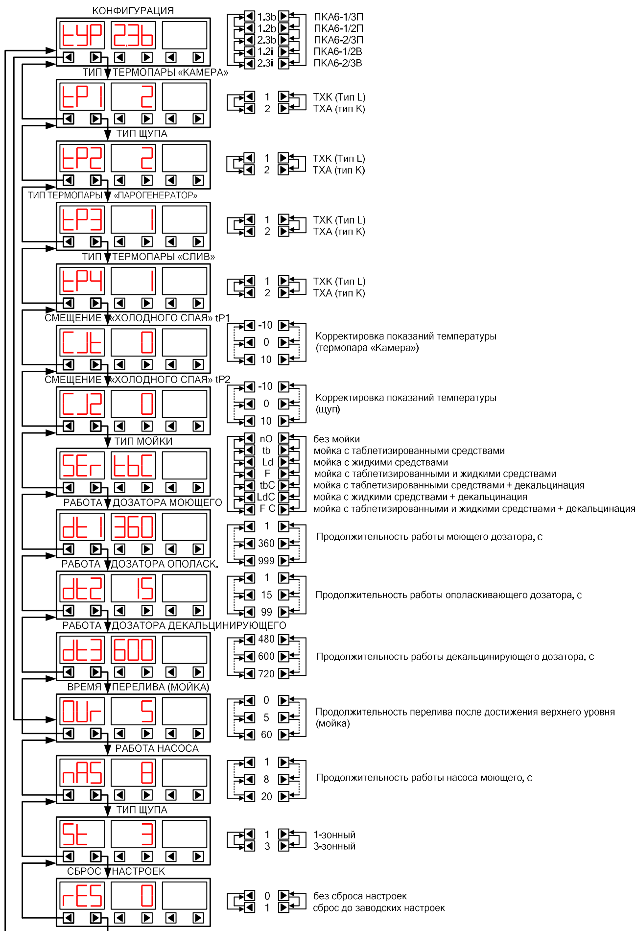
Рис.9. Настройка контроллера
