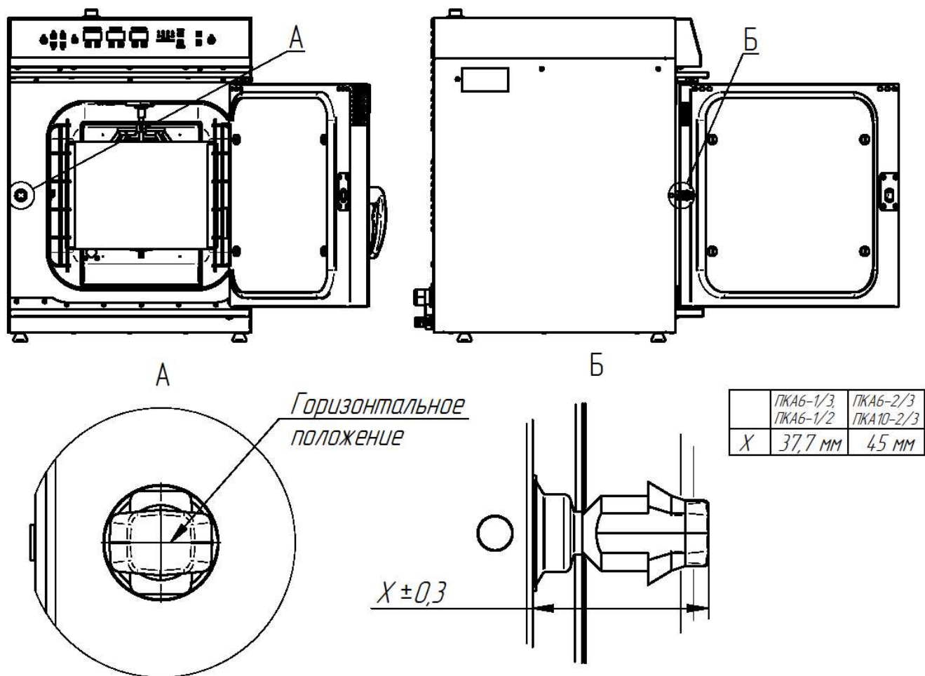
Рис.6. Регулировка замкового устройства
