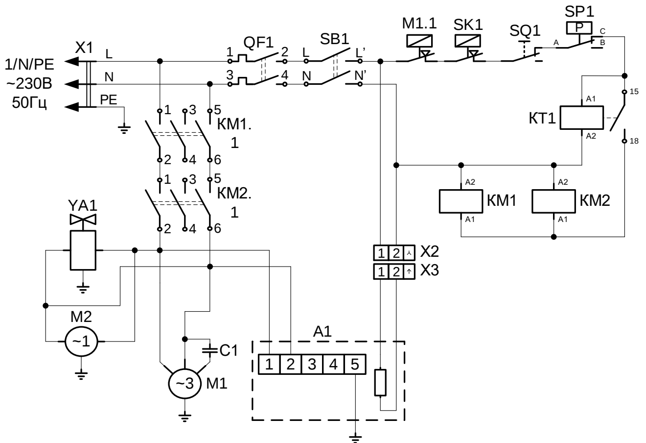
Рис 9. Схема электрическая соединений ЛГ-250Ч-01, ЛГ-400Ч-01
