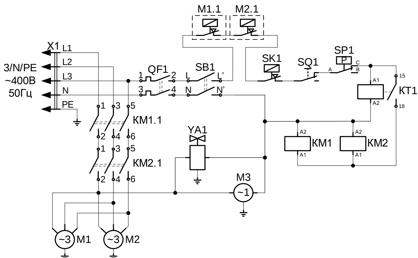
Рис 11. Схема электрическая соединений ЛГ-620Ч-01
