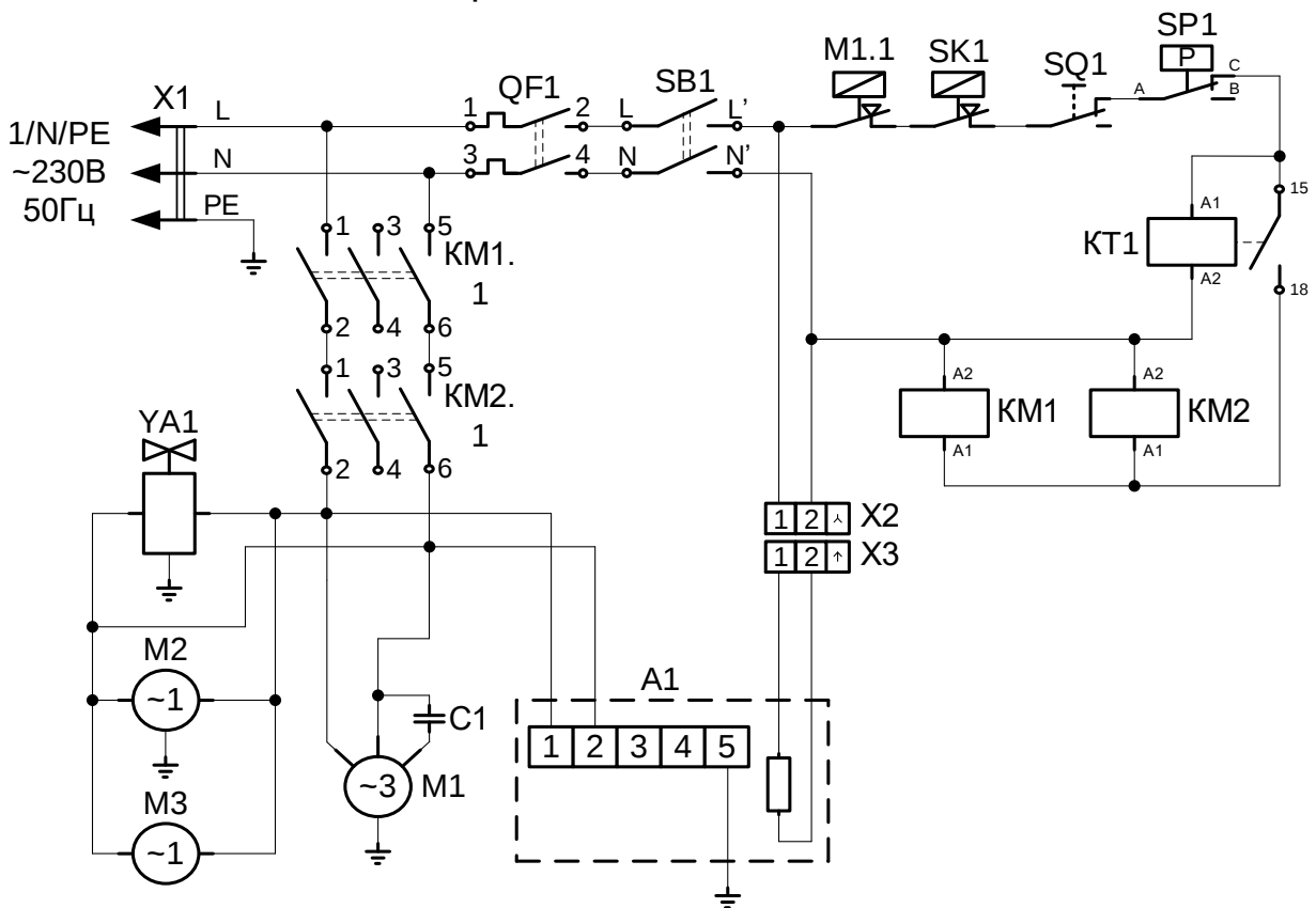
Рис 9. Схема электрическая соединений ЛГ-250Ч-01, ЛГ-400Ч-01
