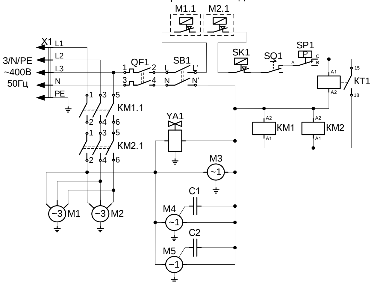
Рис 12. Схема электрическая соединений ЛГ-620Ч-02
