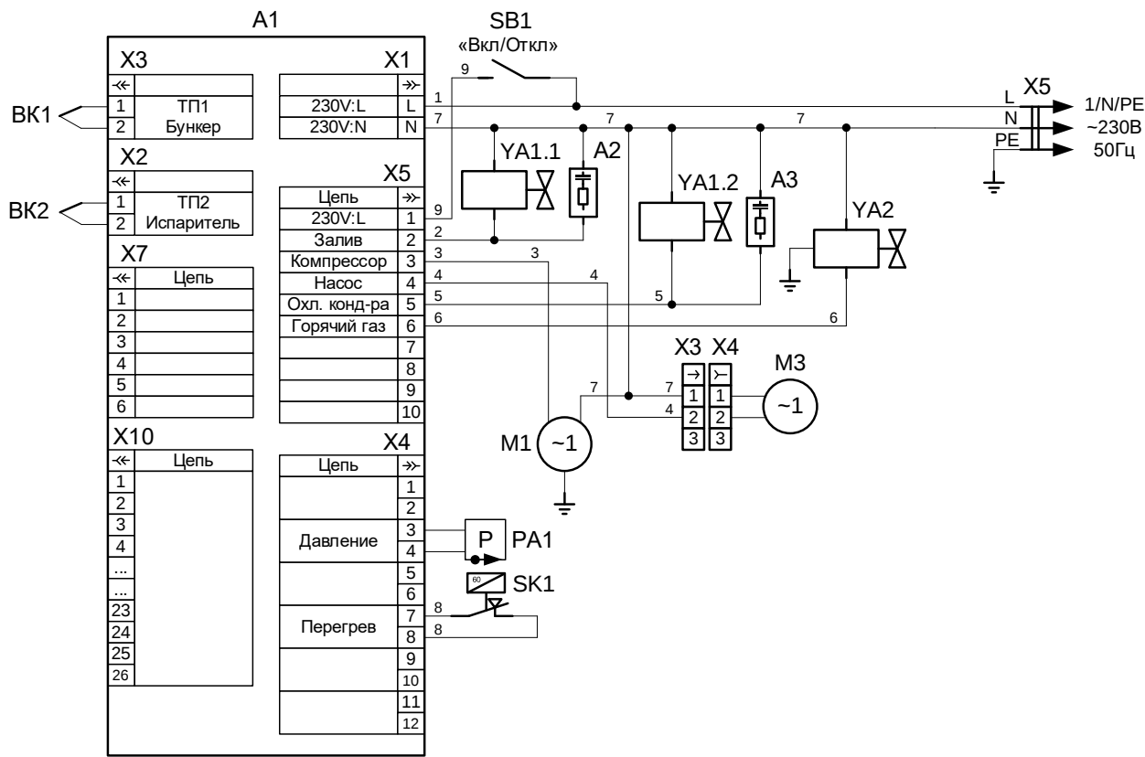
Схема электрическая соединений ЛГ-24/06K-01, ЛГ-24/06K-03
