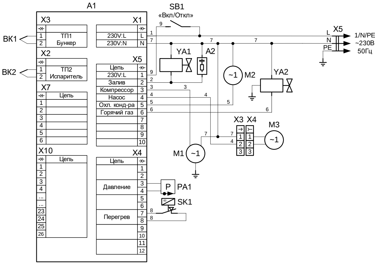
Схема электрическая соединений ЛГ-24/06K-02, ЛГ-24/06K-04
