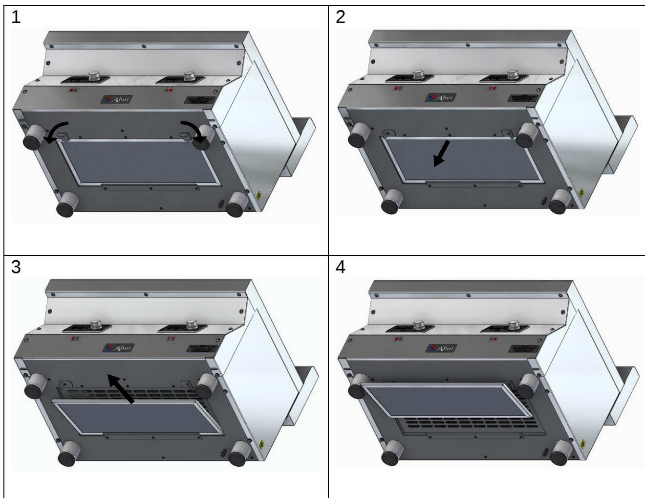
Рис. 8. Извлечение жироулавливающего фильтра
