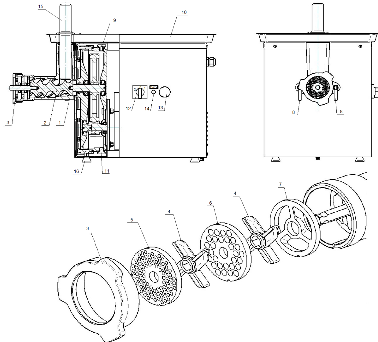
Рисунок 1 Мясорубка МЭП-300
