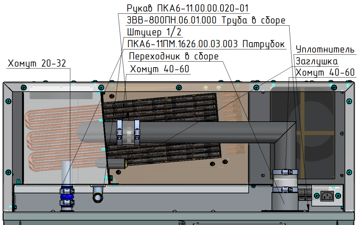
Рис. 1 Подключение зонта к пароконвектому ПА6-11ПМ2
