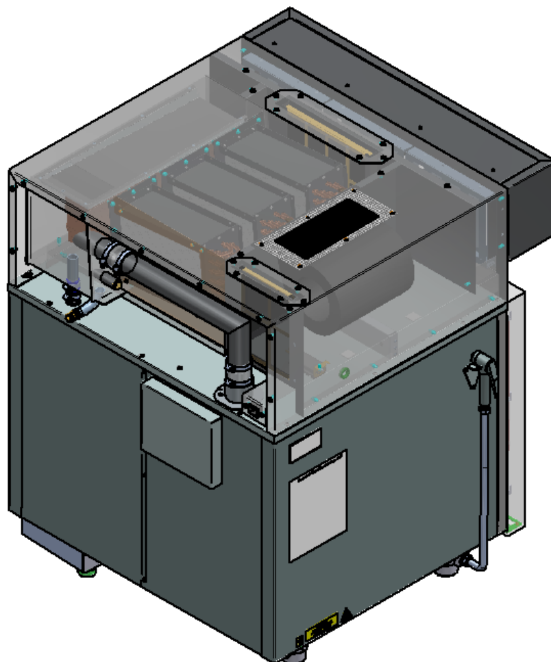
Рис.2 Общй вид зонта с пароконвектоматом
