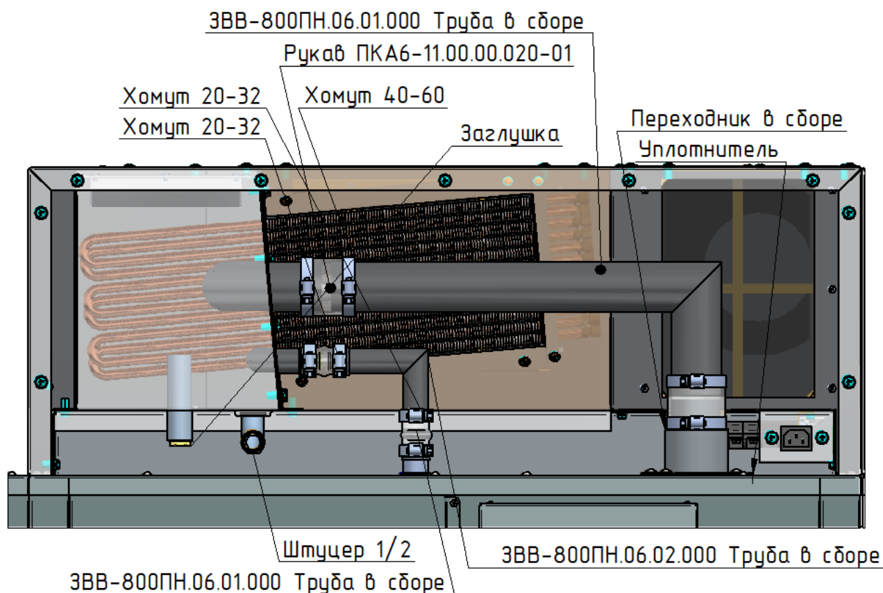
Рис. 3 Подключение зонта к пароконвектомату ПКА6-11ВМ2-01
